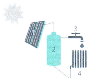
1 Zonnecollector | 2 Opslagvat voor warm water | 3 Tap voor warm water | 4 Radiator voor ruimteverwarming
