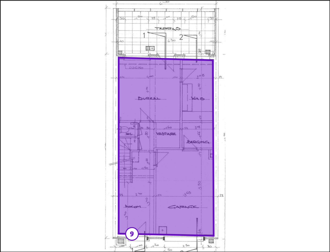
Legende van plan 1.4: Gelijkvloers 0 (vloeren)
